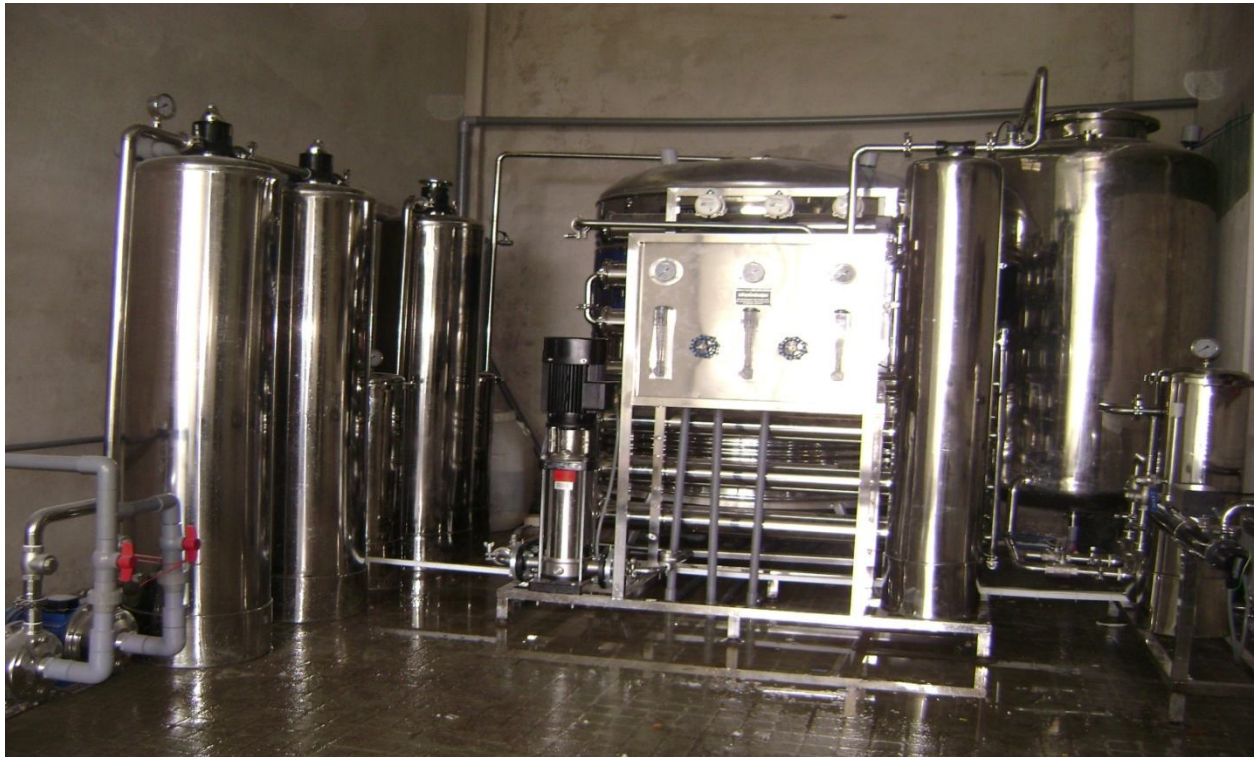
HỆ THỐNG XỬ LÝ NƯỚC RO 2 CẤP 1200 LÍT/H NHÀ MÁY DƯỢC Á CHÂU CẦN THƠ
