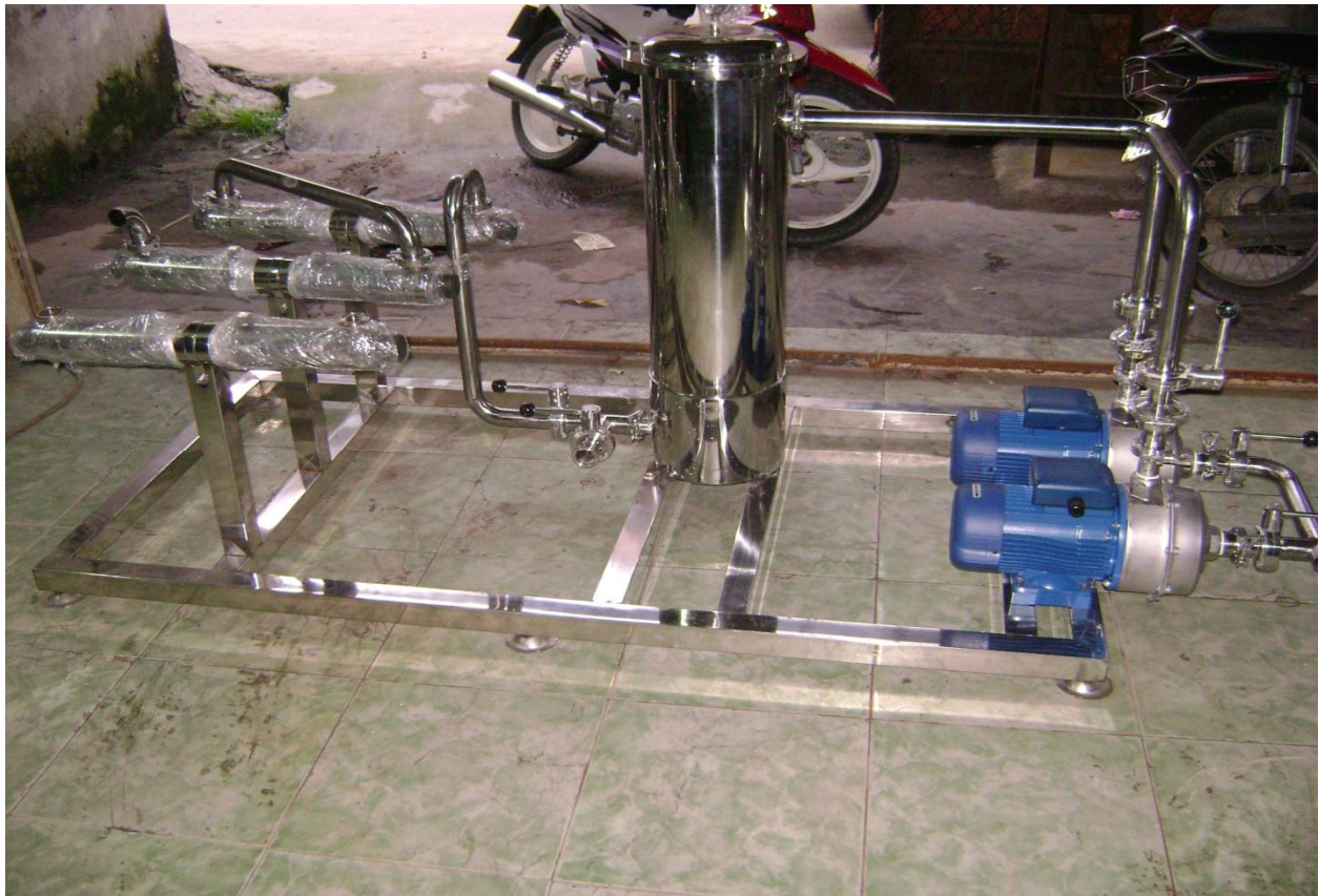
HỆ THỐNG BƠM LỌC 0.2 ĐÈN UV HOÀN LƯU VÀO XƯỞNG SẢN XUẤT NHÀ MÁY DƯỢC PHẨM
